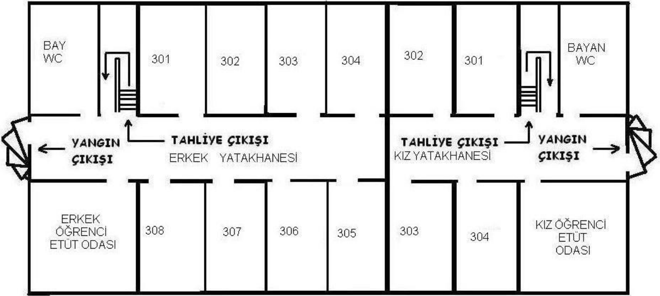
PANSİYON 3.KAT
